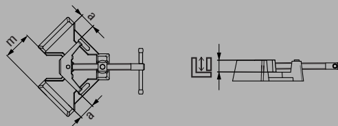
Conjunto de sujeción para soldadura SM 10
