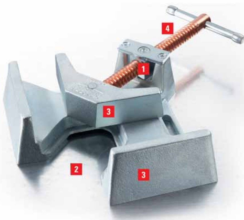
Mordaza para soldadura de ángulos WSM
