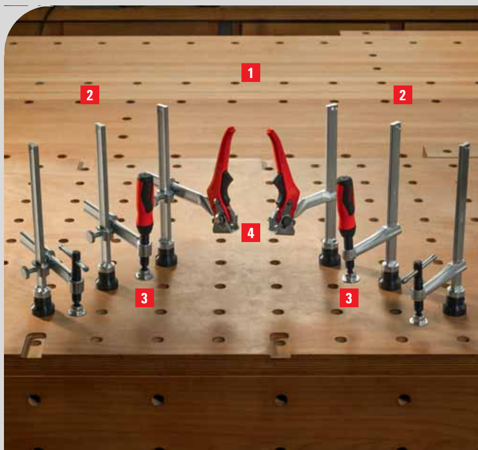
Adaptador para banco de trabajo TW16AW
